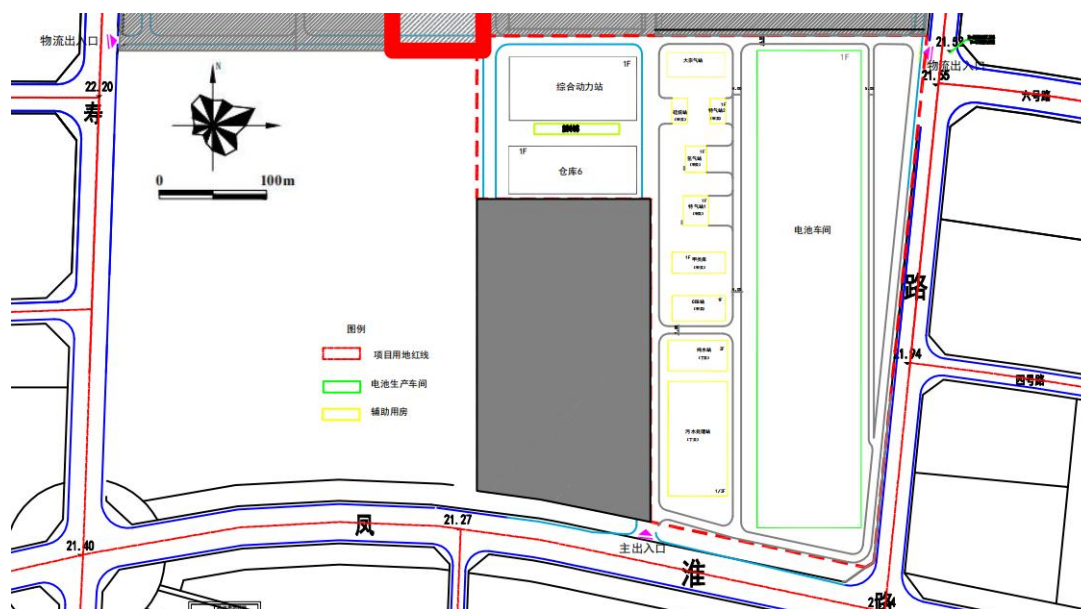
图 2.1-3：项目总平面布置图
